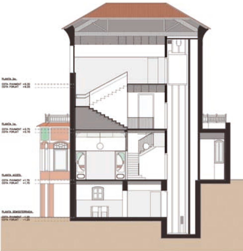
secció transversal
